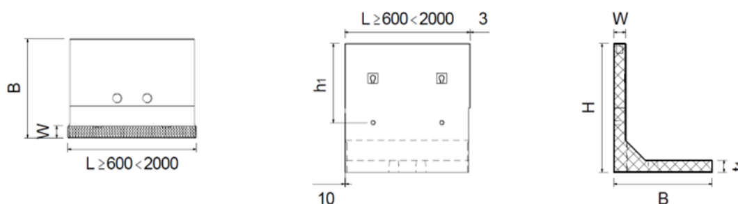
Illustration 9 : Pièce d'ajustement
