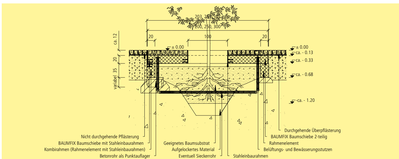
Einbauschema BAUMFIX® Baumscheiben mit Rahmenelement und Überpflästerung (Variante Unterflur)
