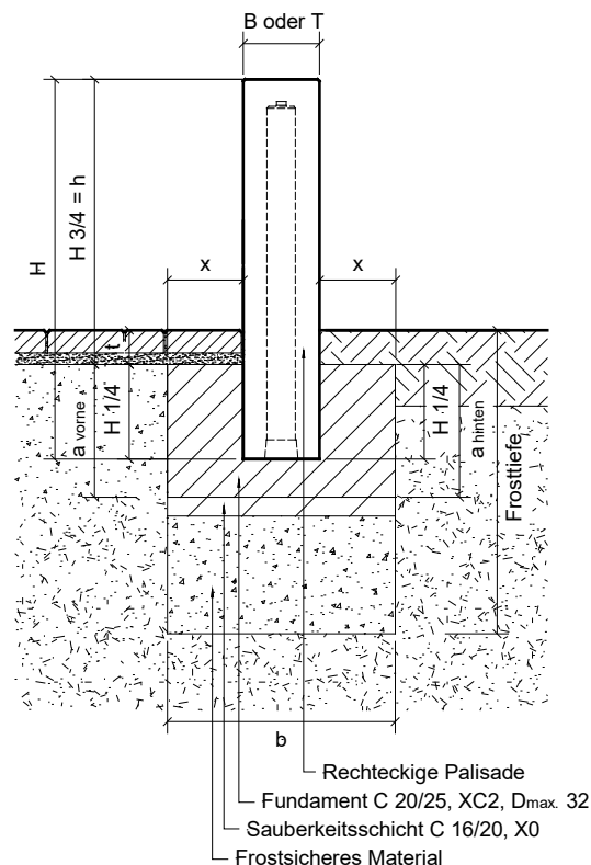
Bild 8: Querschnitt bei freistehenden Palisaden
