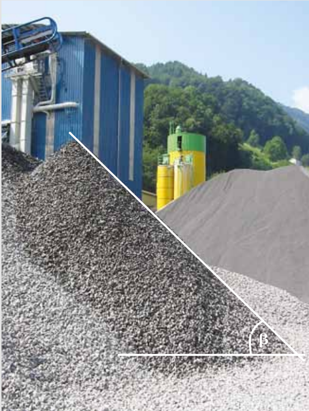
Natürlicher Böschungswinkel \beta
