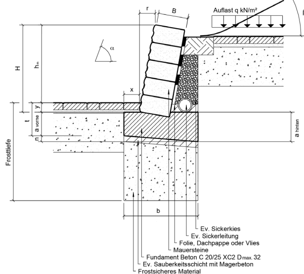
Bild 47: Geneigter Maueraufbau
