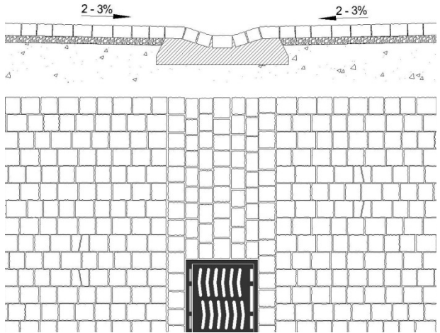
Formation possible de cunettes avec des cunettes en pavés.
