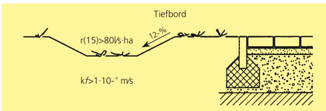
Oberirdisches Abführen des abfliessenden Wassers über Tiefbord
