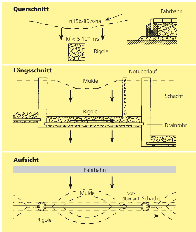
Prinzipskizze Mulden-Rigolen-System
