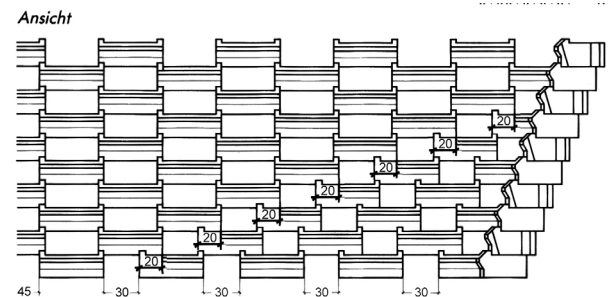
Bild 23: Ansicht Innenecke
