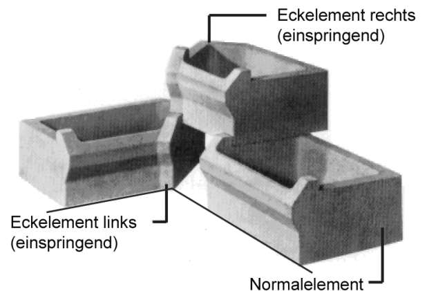
Bild 23: Ansicht Innenecke
