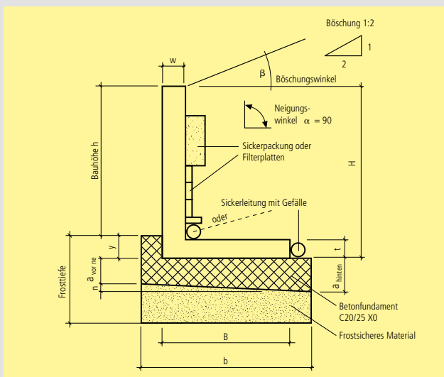
Winkelplatteneinbau
