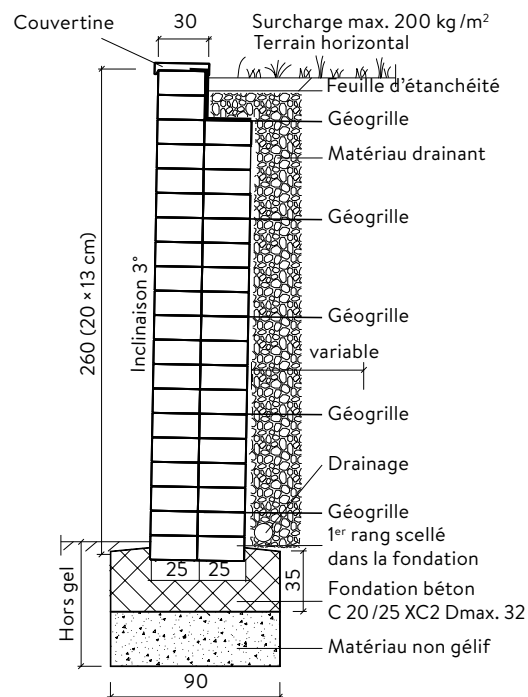
Exemple de réalisation d'un mur avec une armature en géogrid, épaisseur = 50 cm
