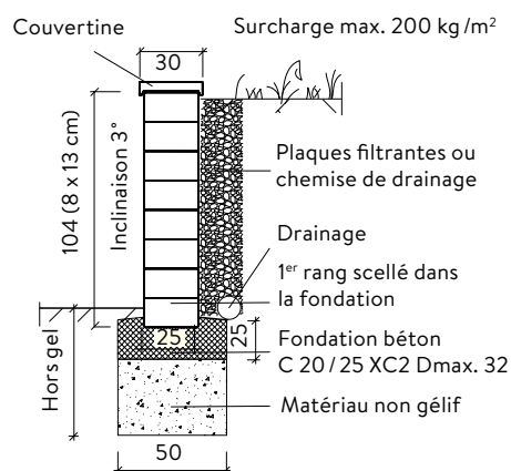
Exemple de réalisation d'un mur sans géogridle, épaisseur = 25 cm
