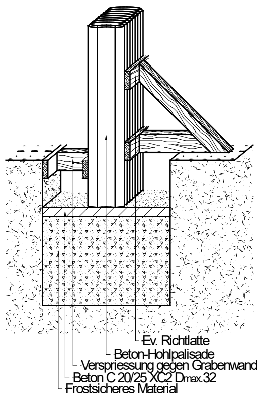
Bild 14: Einbau Palisaden
