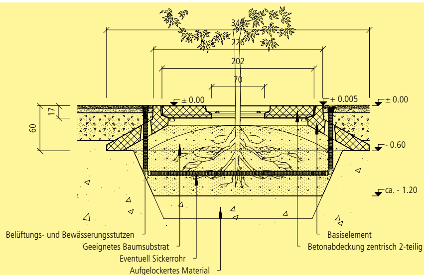
Einbaueschema COPAL CUPOLA Baumwurzelraumschutz mit Betonabdeckung zentrisch
