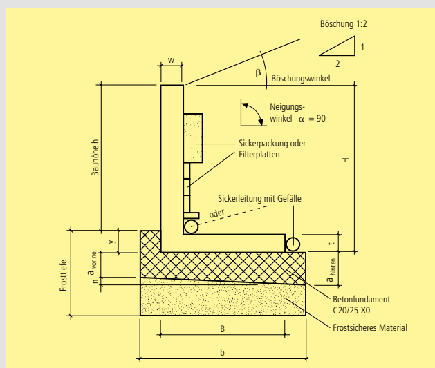
Winkelplatteneinbau
