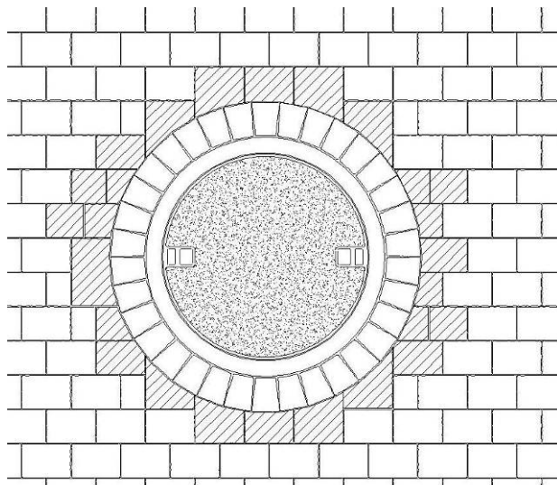
Bild 30: Optimales Verlegebild bei Schachtabanschlüssen, schraffierte Steine zeigen die zugeschnittenen Passsteine
