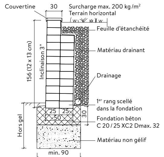
Exemple de réalisation d'un mur sans géo grille, épaisseur = 50 cm
