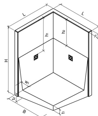
Bild 11: ROZTEC® MIDI ECKEelement Typ 2
