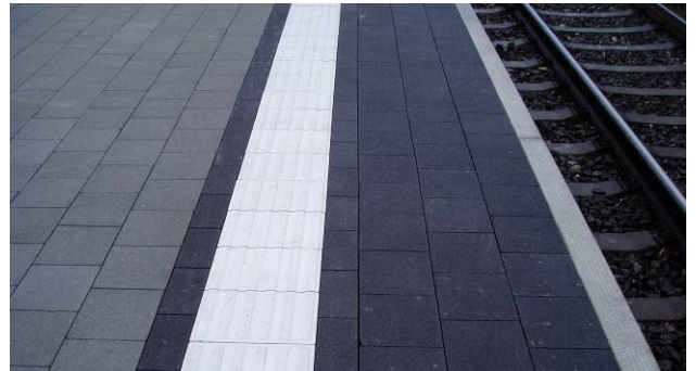
Bild 19: Anordnung von CARENA® Pflastersteinen mit Oberflächenfarbe anthrazit
