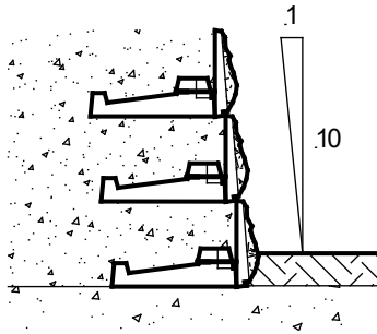
Bild 27: Wandneigung 1:10 (84°), Standard
