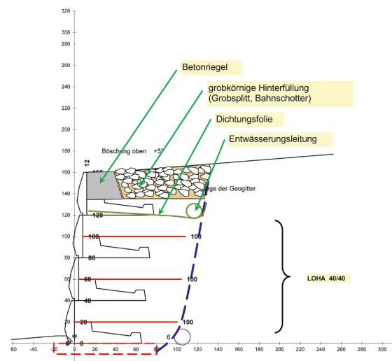
Diagramm 1: Dichtungsfolie und Entwässerungsleitung unterhalb des Grobsplittes oder Bahnschottes
