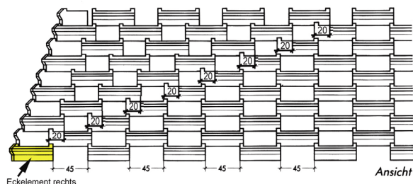
Bild 20: Ansicht Aussenecke
