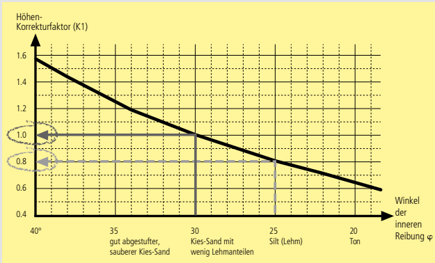
Korrekturfaktor (K1) für Mauerhöhen beeinflusst durch den inneren Reibungswinkel \varphi des Bodennaterials. Darstellung 6
