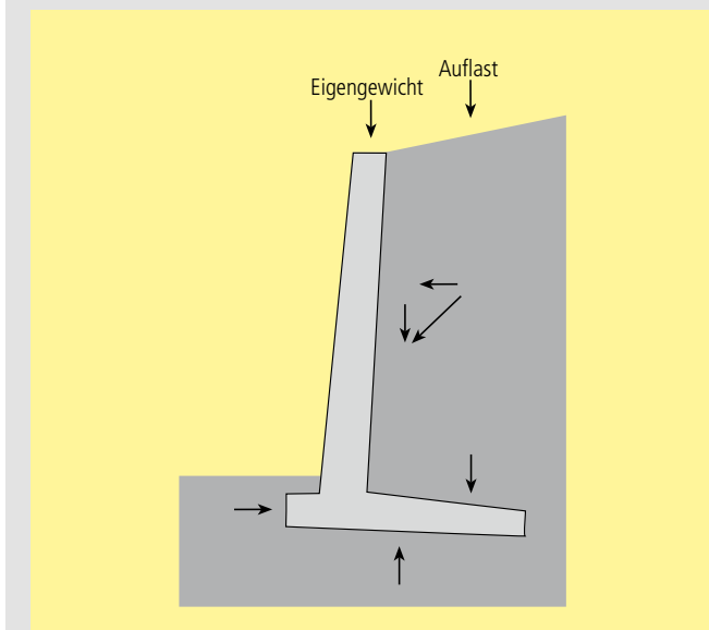
Winkelstützmauer
