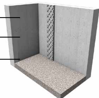
Coupe schématique Sortie amphibie AMFIX® intégrée dans un bassin de rétention
