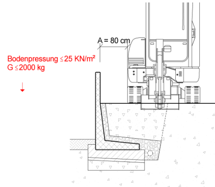
Bild 18: Lastfall G
