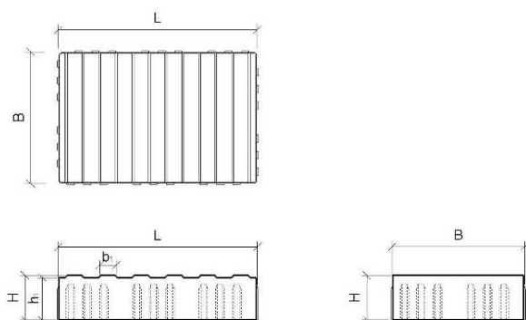
Bild 5: CARENA® Sicherheitslinienstein Typ N; H 8 cm
