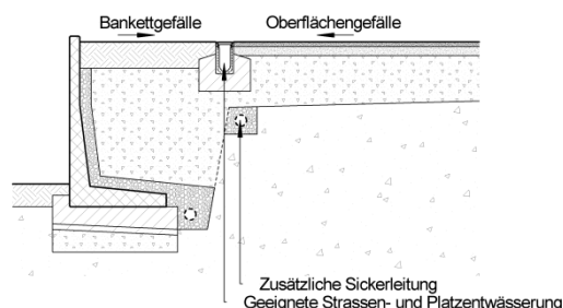
Bild 29: Zusätzliche Entwässerung
