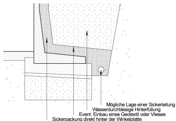
Bild 28: Mögliche Lage einer Sickerleitung
