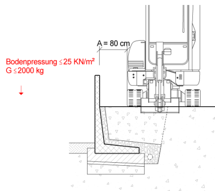
Bild 18: Lastfall G
