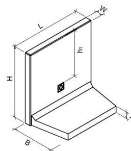
Bild 5: ROZTEC® MIDI Winkelplatte Typ 1
