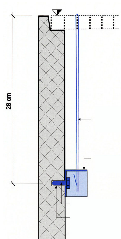
Bild 15: Einbruchsicherung
