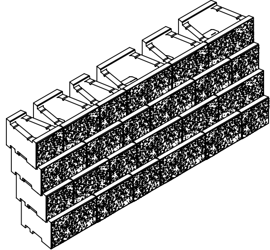
Bild 10: Isometrie Verlegemuster 2
