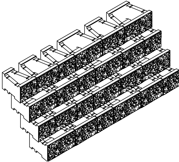
Bild 9: Isometrie, Verlegemuster 1
