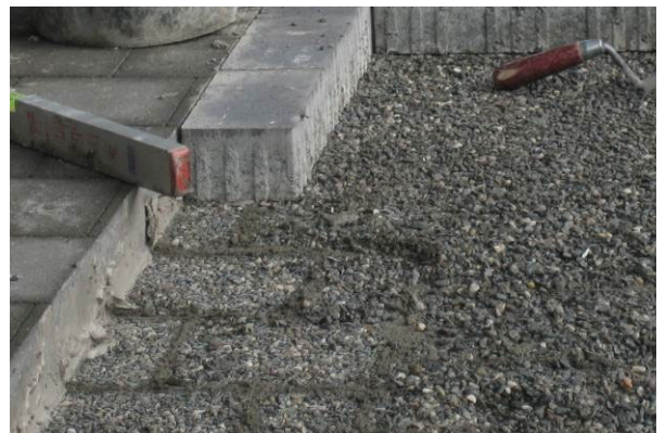
Bild 33: Instandsetzung der Bettungsschicht
