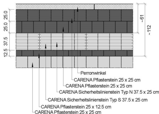
Bild 8: Anordnung als Beispiel bei Durchfahrtsgeschwindigkeiten V_R 101 bis 120 km/h oder V_A 91 bis 100 km/h ( b \sim 61 cm) bei der Verwendung von CARENA® Pflastersteinen H = 8 cm
