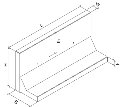
Bild 5: Winkelplatte
