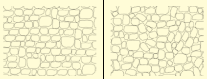
Verlegemuster Römischer Verband Wilder Verband
