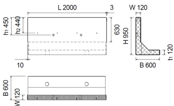
Bild 5: Perronwinkel Typ 5
