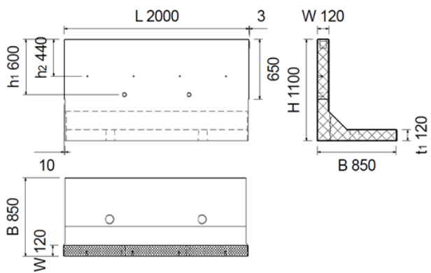
Bild 3: Perronwinkel Typ 3 (Standardtyp für Schmalspurbahn)
