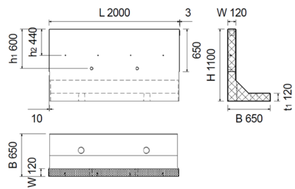
Bild 4: Perronwinkel Typ 4 (Standardtyp für Schmalspurbahn)
