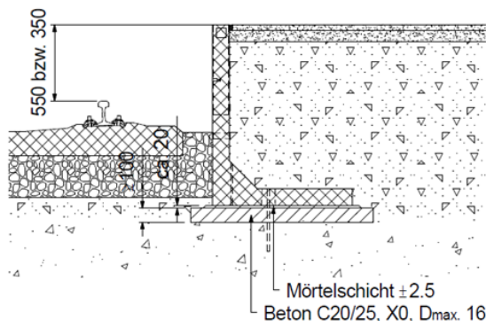
Bild 11: Perronwinkel - Standardprofil
