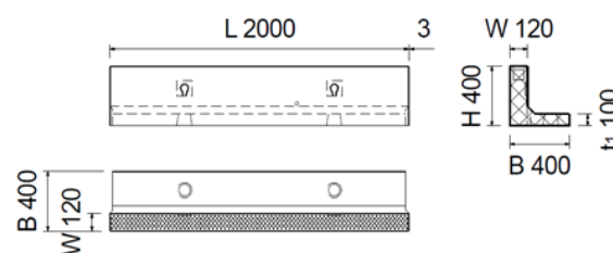
Bild 8: Perronwinkel Typ 8
