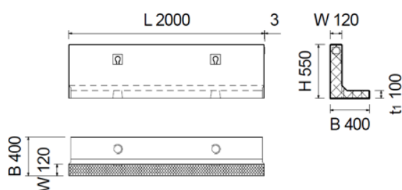
Bild 7: Perronwinkel Typ 7
