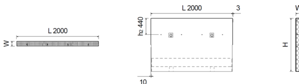
Bild 10: Wandplatten
