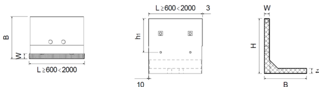
Bild 9: Passtück
