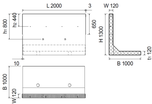
Bild 1: Perronwinkel Typ 1 (Standardtyp für Normalspurbahn)
