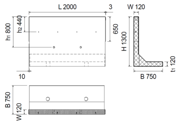
Bild 2: Perronwinkel Typ 2 (Standardtyp für Normalspurbahn)
