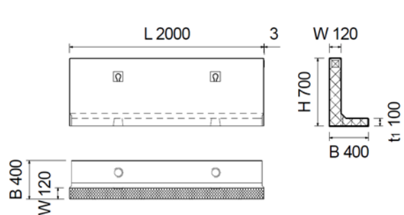
Bild 6: Perronwinkel Typ 6
