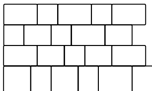
Verlegemuster 1 Reihenverband, Randabschluss zuschneiden
