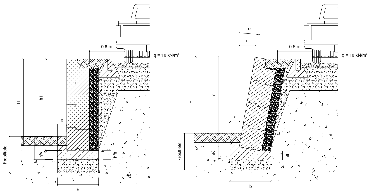
Bild 29 Streifenfundamentabmessungen für Lastfall C
