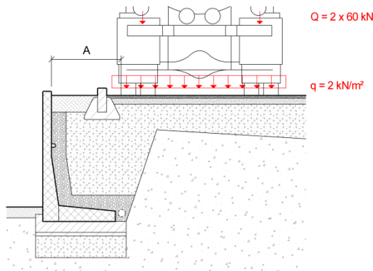
Bild 13: Lastfall C4
