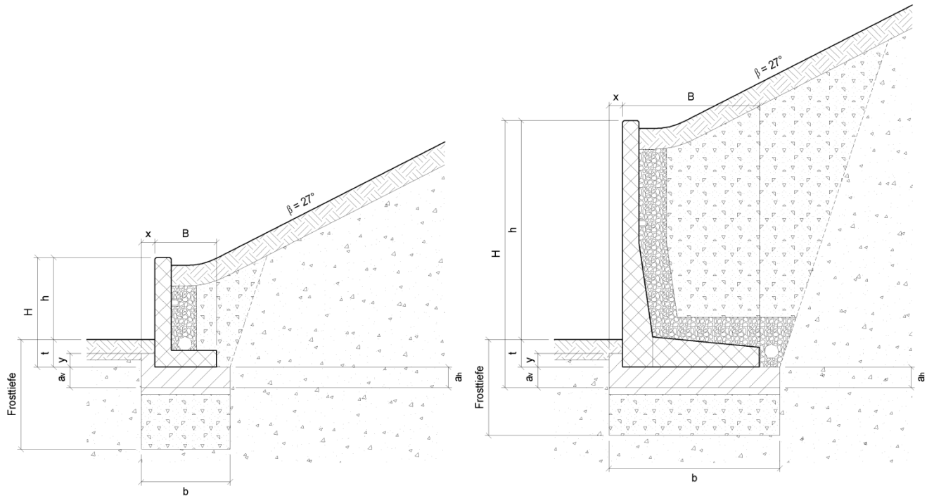
Bild 42: Fundamentabmessungen für Lastfall E, 1:2, \beta = 27^\circ
