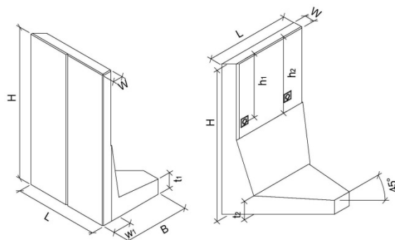
Bild 10: COMOFORTE® Eckelemente Typ 2
