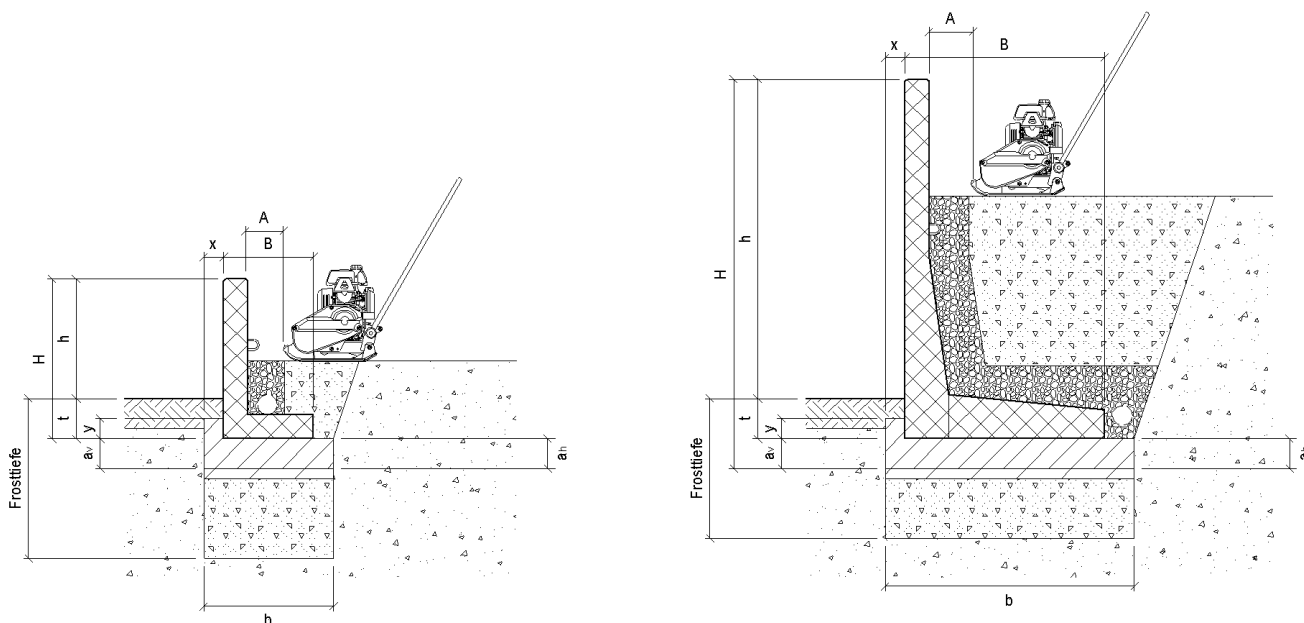
Bild 43: Fundamentabmessungen für Lastfall F2, A = 20 cm
