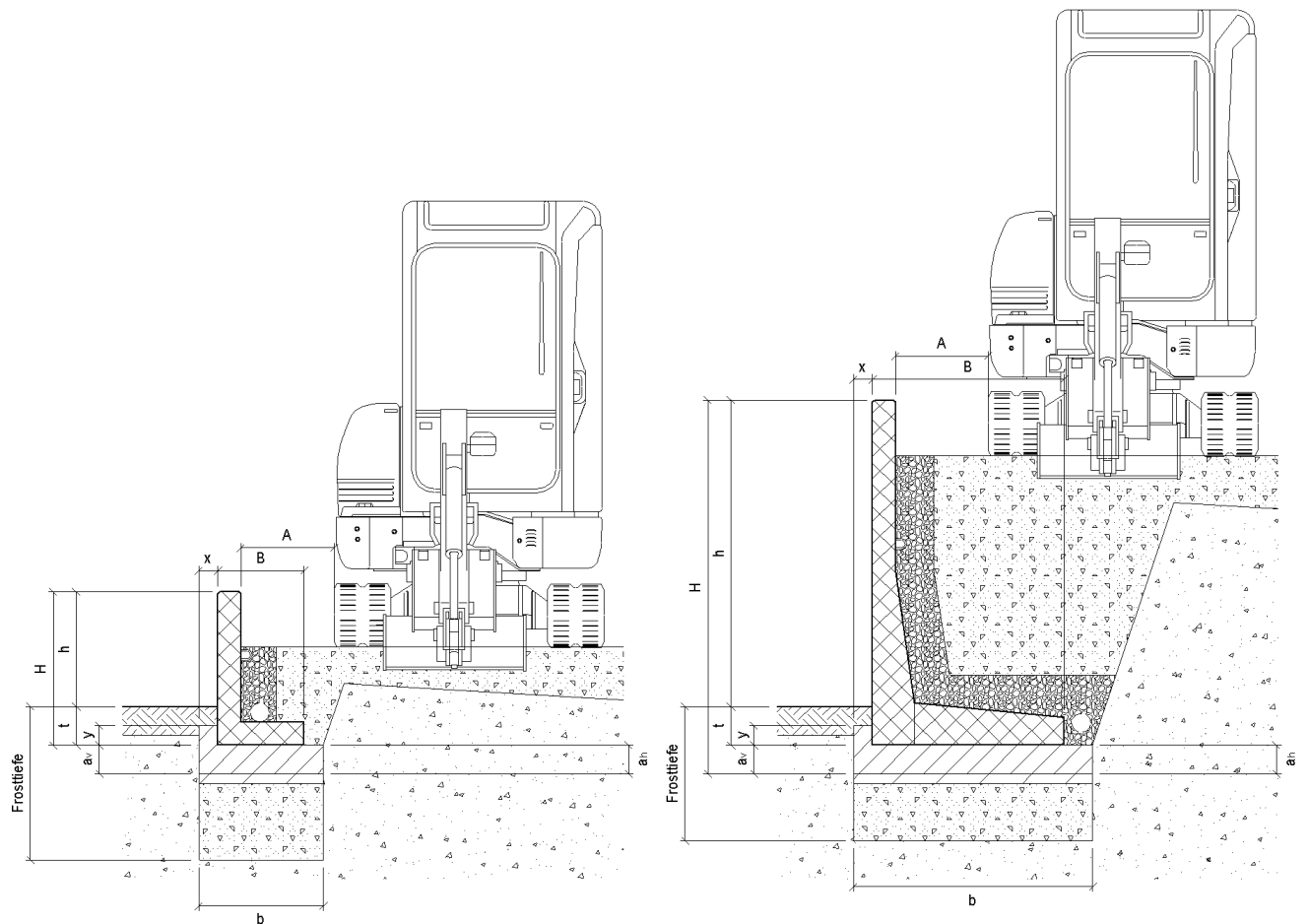
Bild 44: Fundamentabmessungen für Lastfall G, A = 80 cm
