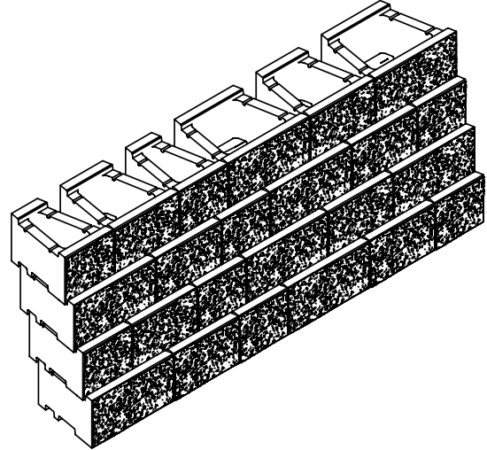
Bild 10: Isometrie Verlegemuster 2
