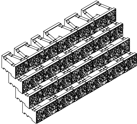
Bild 9: Isometrie, Verlegemuster 1
