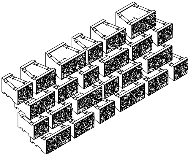
Bild 11: Isometrie Verlegemuster 3
