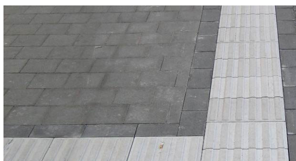
Bild 29: Ideale Anordnung von Passsteinen bei einem Anschluss an eine Sicherheitslinie
