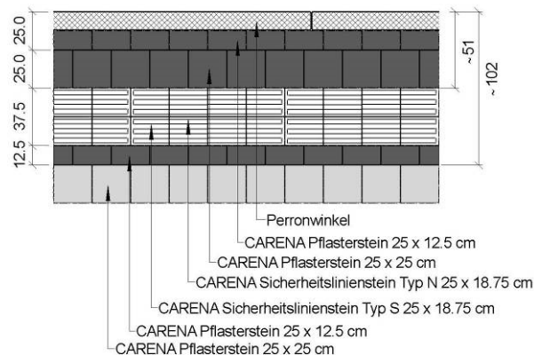
Bild 9: Anordnung als Beispiel bei Durchfahrtsgeschwindigkeiten V_R bis 100 km/h oder V_A bis 90 km/h ( b \sim 51 cm) bei der Verwendung von CARENA® Pflastersteinen H = 6 cm
