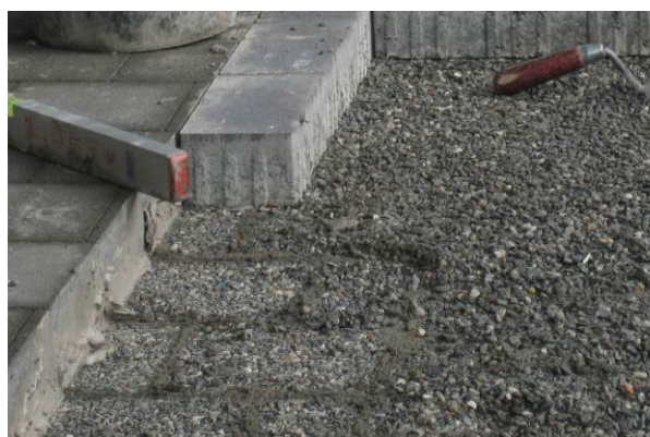
Bild 33: Instandsetzung der Bettungsschicht
