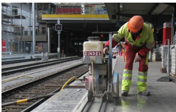
Bild 31: Einsatz einer kleinen Belagsfräse
