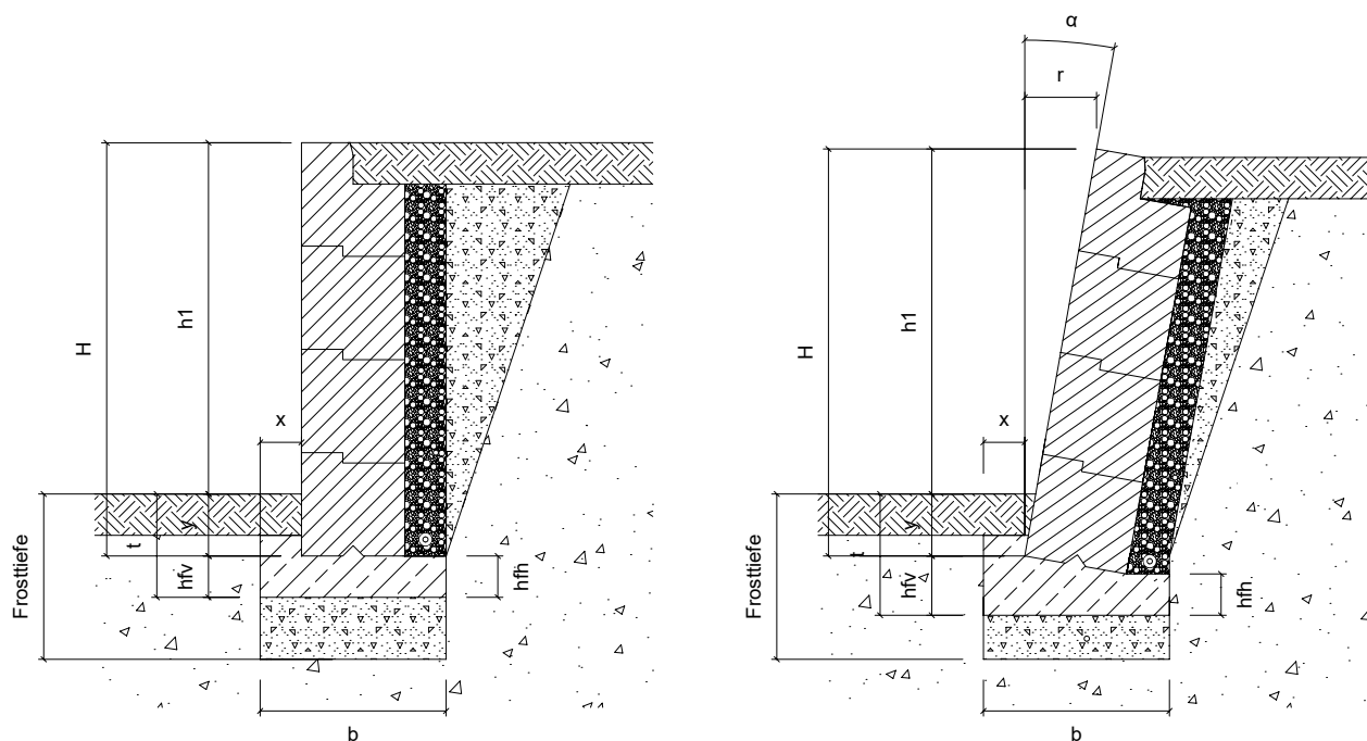
Bild 27 Streifenfundamentabmessungen für Lastfall A
