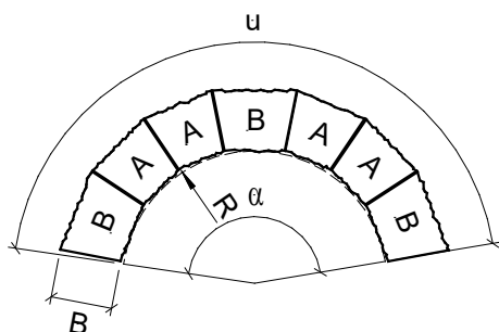
Bild 31: Optimale Muffenbildung
