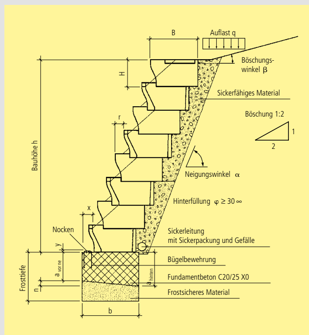
Böschungselemente Aufbau
