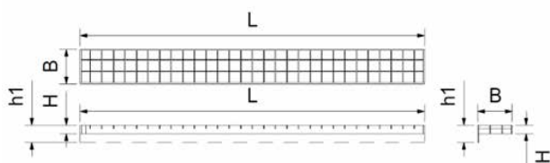
Bild 2: Schematische Darstellung der Gitterrost 100
