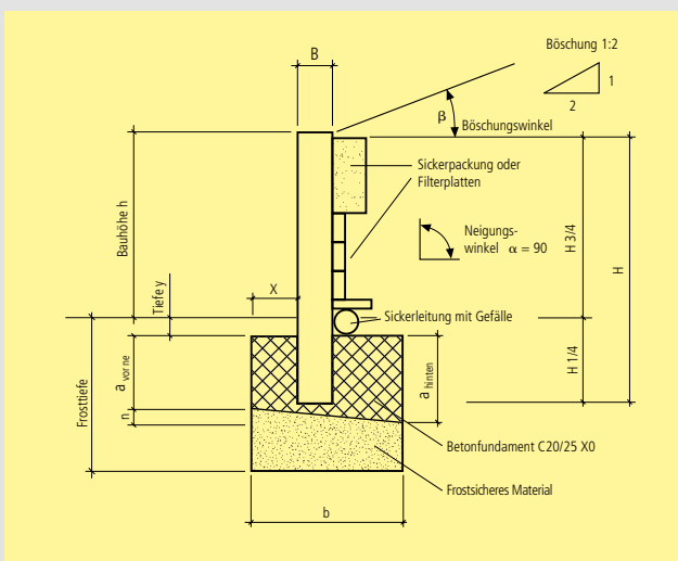
Palisadeneinbau
