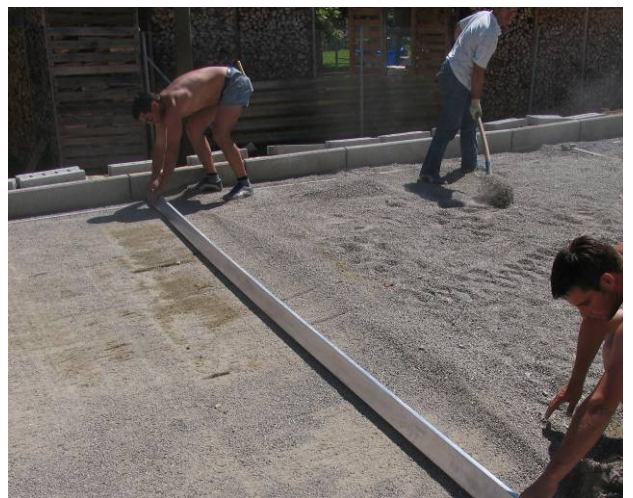
Bild 33: Abziehen der Bettungsschicht
