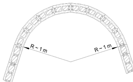
Bild 29: Schematische Darstellung bei der Verwendung von Radiusspaltsteinen
