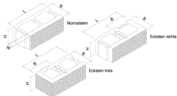
Bild 7: Spaltsteine, 1-seitig gespalten
