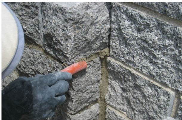
Bild 47: Modellieren der Fuge mit einem Kunststoffrohr
