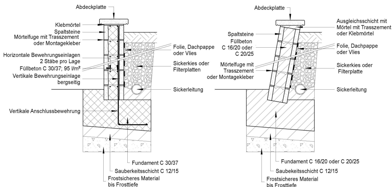
Bild 28: Darstellung des Aufbauquerschnittes
