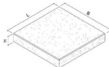
Bild 19: Abdeckplatten, gefast, bewehrt
