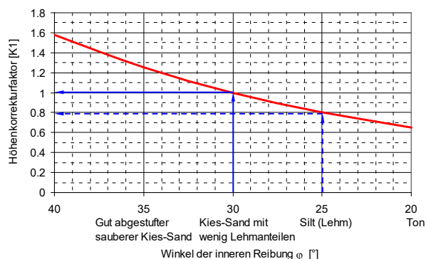
Diagramm 1: Höhenkorrekturfaktor K1 bei Änderung der Bodenkennwerte
