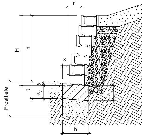
Bild 28: Lastfall D, Rücksprung 5,5 cm, \alpha = 76^\circ
