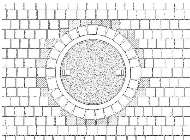
Mögliches Verlegebild bei Schachtanschlüssen. Schraffierte Steine zeigen die zugeschnittenen Passsteine an.
