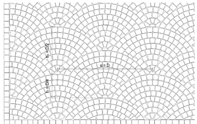
Schuppenplasterung mit FRIEDA® Pflastersteinen
