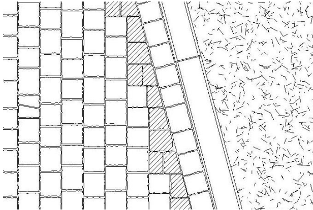
Mögliches Verlegebild beim Anschluss von schräg verlaufenden Abschlüssen. Schraffierte Steine zeigen die zugeschnittenen Passsteine an.
