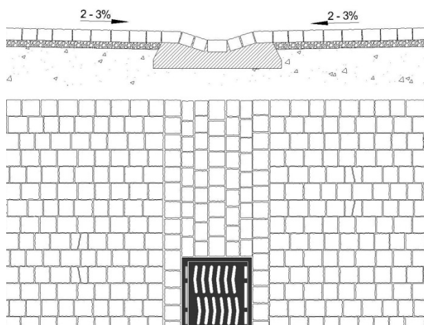
Mögliche Rinnenausbildung mit FRIEDA® Pflastersteinen
