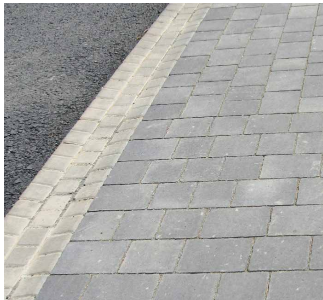
Mögliche Rinnenausbildung mit Pflasterrinnen.
