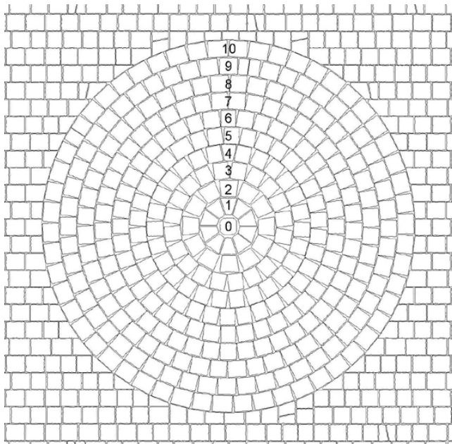
Kreisplasterung mit FRIEDA® Pflastersteinen
