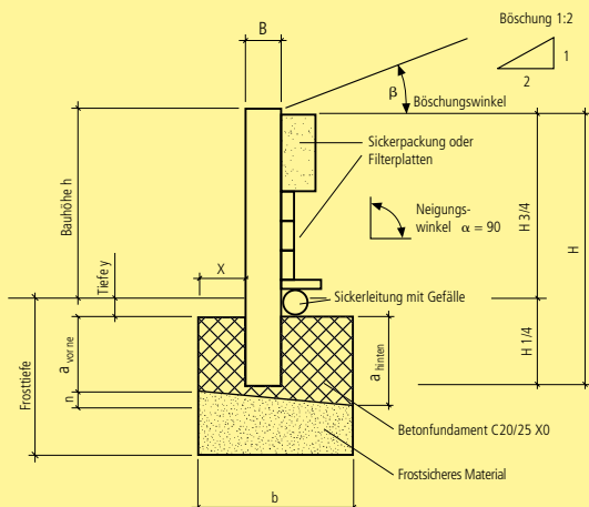
Palisadeneinbau
