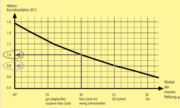
Korrekturfaktor (K1) für Mauerhöhen beeinflusst durch den inneren Reibungswinkel \varphi des Bodenmaterials.
