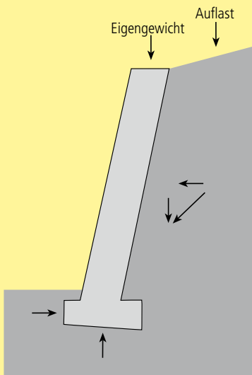
Schwergewichtsmauer
